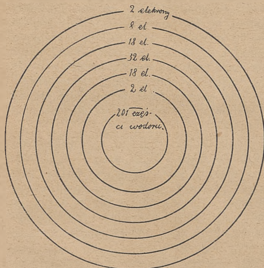
Schemat budowy atomu rtęci i złota. — Ciężar atomowy rtęci jest 201 (cyfra zaokrąglona). Ciężar złota: 197. Po odrzuceniu z atomu rtęci jednej cz. alfa (ciężar 4) pozostaje atom o ciężarze złota. Pozatem atom rtęci posiada 80 elektronów, po usunięciu jednego elektronu z ostatniego koła pozostanie ich 79, czyli tyle ile ich posiada złoto
