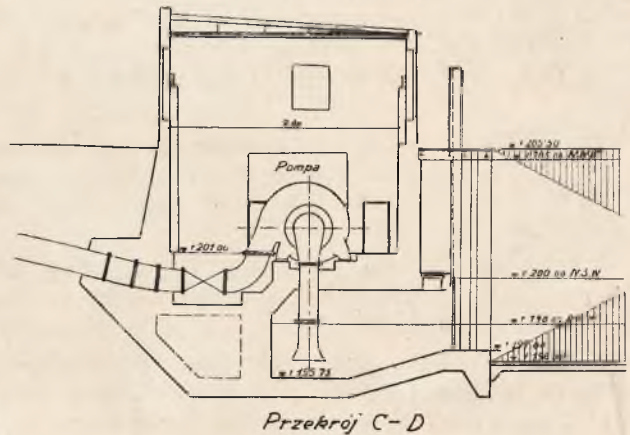
Sifownia zbiornikowa na Bielcach
