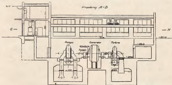
Sifownia zbiornikowa na Bielcach
