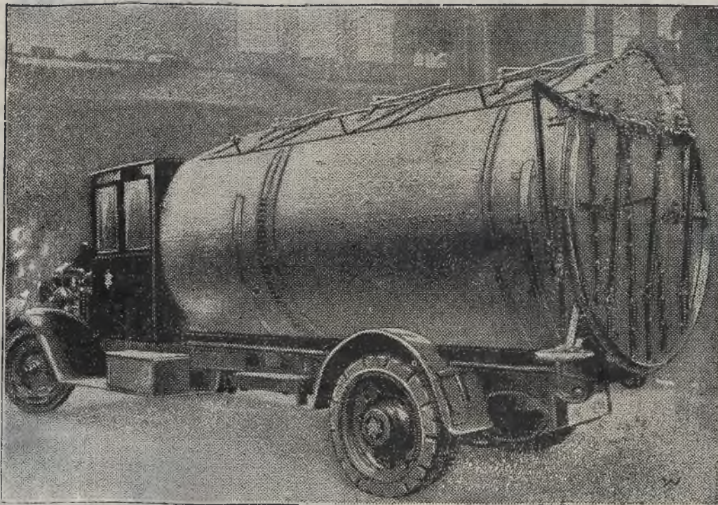
RYCINA POGLĄDOWA. Automobilowy wóz do śmieci, skośnie od tyłu widziany. Do nasypywania śmieci okręca się kociel za pomocą kół zębitych, tak że śmieci można wygodnie wrzucić. Do wyładowania unosi się kociel z przodu w górę a zatrząsk w tyłu otwiera i samoczynnie kociel wypróżnia.
