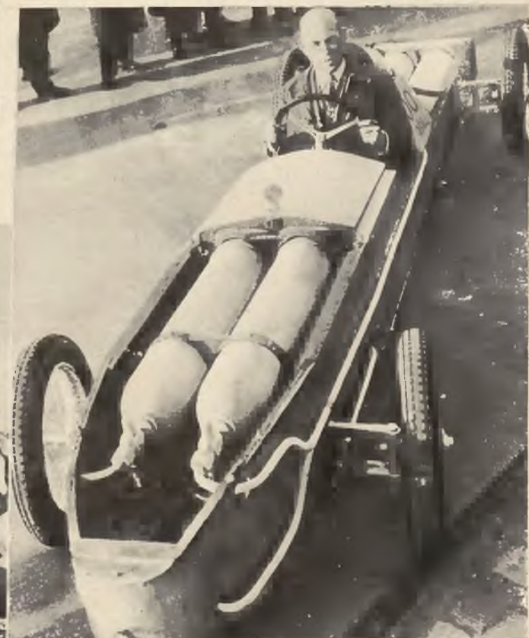
Nowy model wozu raketowego, który zademonstrował twórca Max Valier na torze Avus w Berlinie.
