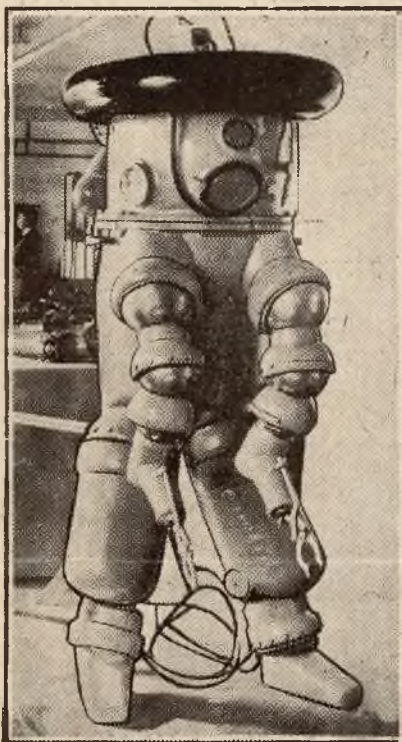
W poszukiwaniu angielskiej łodzi podwodnej „M. 1.” Nurek niemiecki w najnowszym aparacie, pozwalającym na zanurzenie się do 150 m. pod powierzchnię morza.
