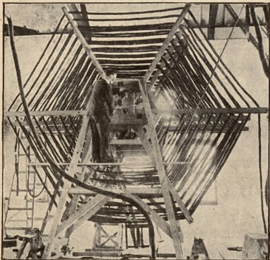
Największa radjostacja świata w Hillmorton. Robotnicy montują olbrzymią cewkę indukcyjną o wadze kilkuset kilogramów.
