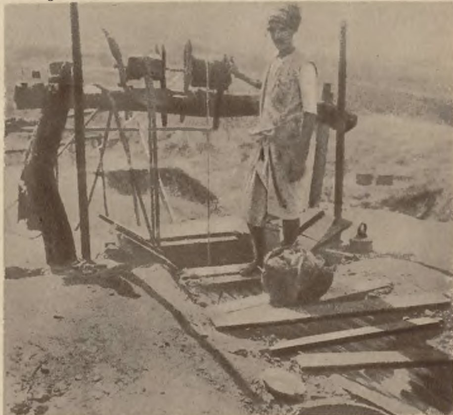
Prymitywne dobywanie olejów ziemnych w Burmie. Ze źródeł 100 metrowej głębokości czerpią krajowcy cenny olej za pomocą dwu małych wiader.
