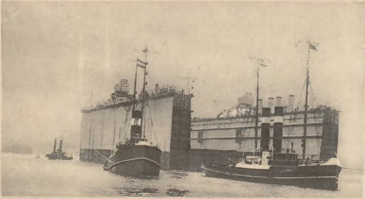
Olbrzymie doki pływające zbudowane w Anglii, opuszczają Tynemouth udając się do Singapore, gdzie mają służyć dla budowy okrętów admiralicji angielskiej.
