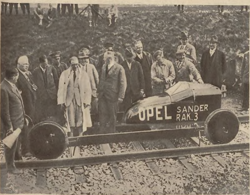
Na linii kolejowej Burgwedel-Celle odbyły się nowe próby wozu raketowego Opla, na szynach. Przy pierwszej udanej próbie osiągnięto 254 km. na godzinę przy drugiej próbie która miała być 4 razy silniejsza, wóz się spalił. Na lewo wóz „Opel Rak III“ (w białym płaszczu inż. Opel). Na prawo wóz w pełnej jeździe.
