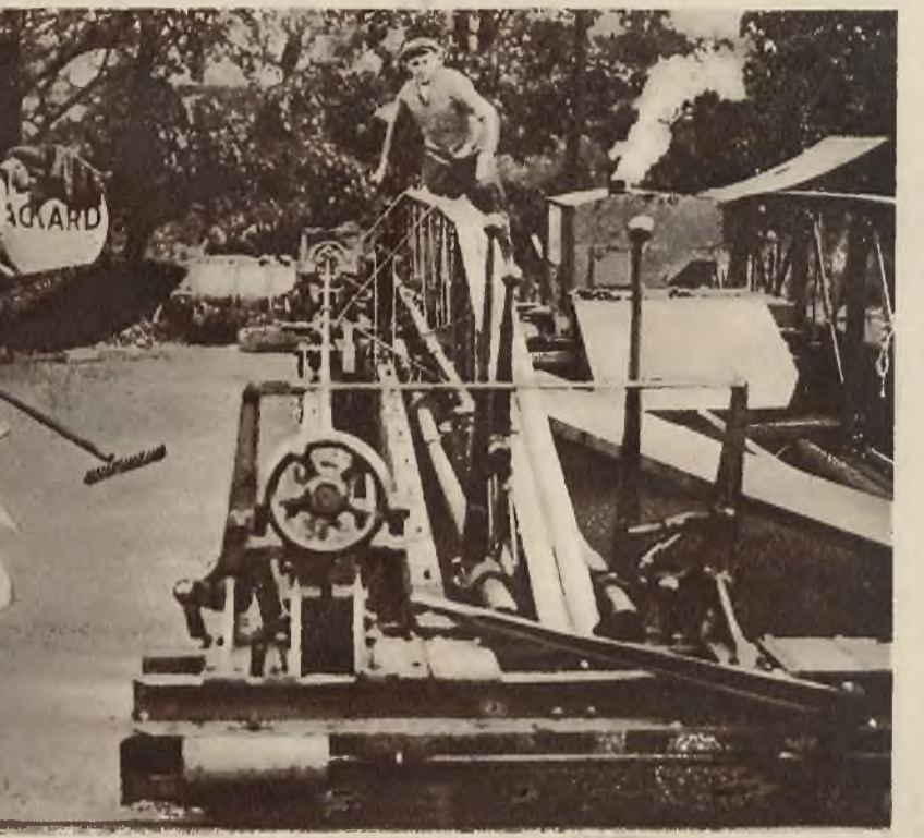
Świeżo wprowadzona w użytek maszyna do asfaltowania i naprawiania ulic.
