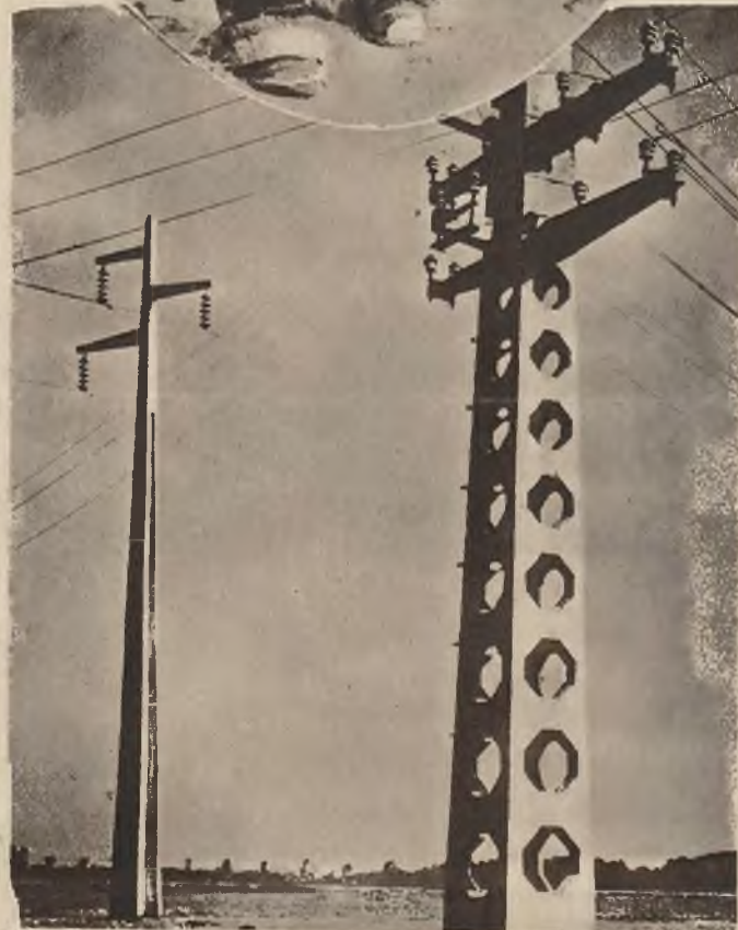
Nowe modele słupów telegraficznych — zrobione są one z betonu i odznaczają się estetycznym wyglądem.
