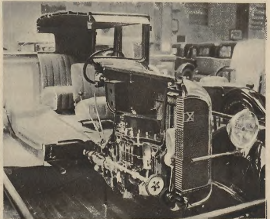
Przekrój samochodu marki Citroen na wystawie samochodów w Berlinie, na którym można rozpoznać system motoru.
