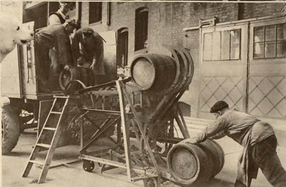
Jeden z browarów berlińskich wprowadził praktyczną nowość; maszynę do podnosze- nia beczek, elektrycznie popędzaną.
