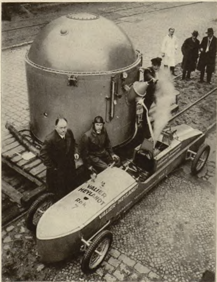
Zdjęcia z próbnej jazdy (na prawo) nowego wozu rakietowego inż. Valier. U góry napełnianie wozu płynami popędowymi. Wóz ten nie jest poruszany jak dotychczasowe siłą eksplodujących rakiet, ale siłą rzutu wstecznego mieszanki gazowej wytwarzanej w wozie.
