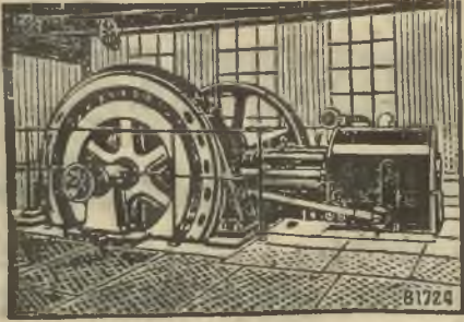
Lokomobila wentylowa o parze przegrzanej z dynamicznym bezpośrednim połączeniem.
