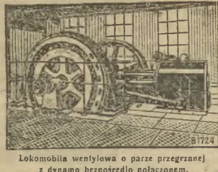
Lokomobila wentylowa o parze przegrzanej z dynamo bezpośrednio połączonym.
