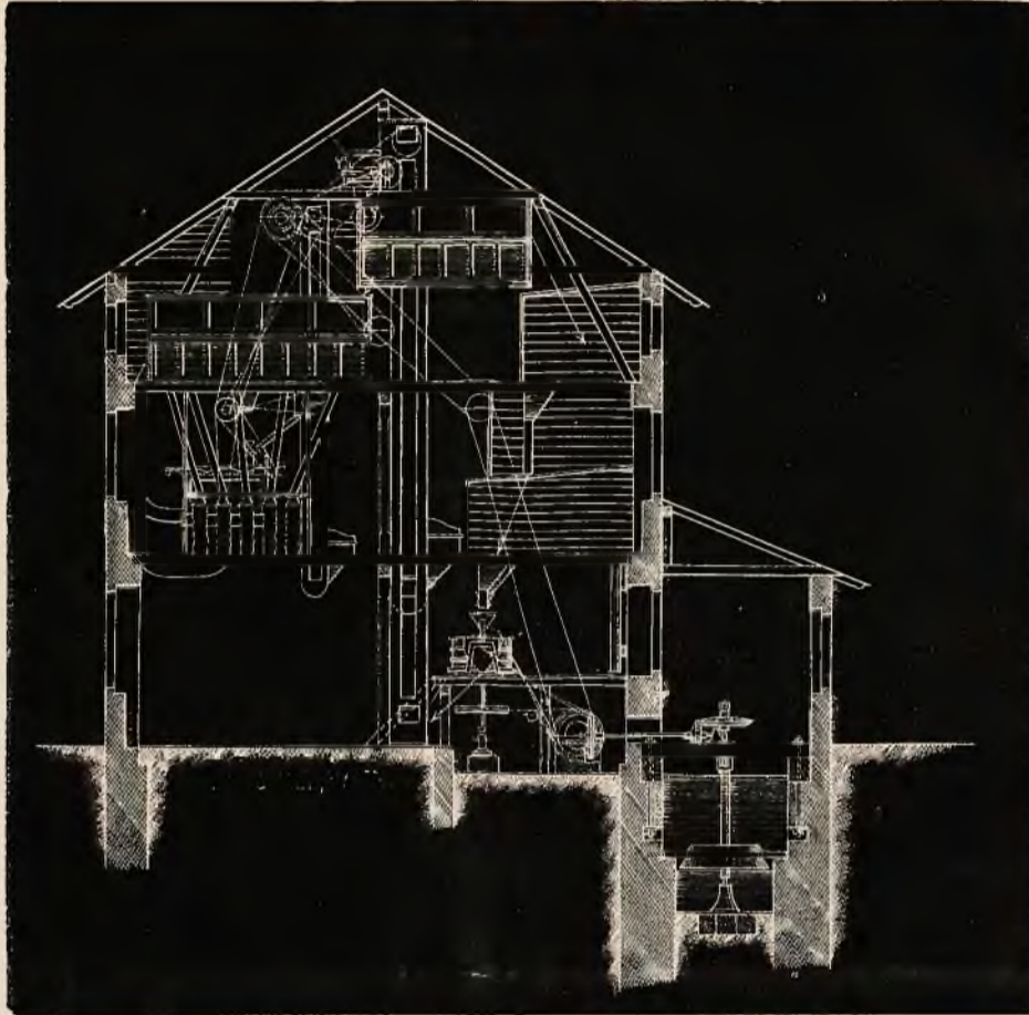
Przekrój poprzeczny (ryc. 5)
