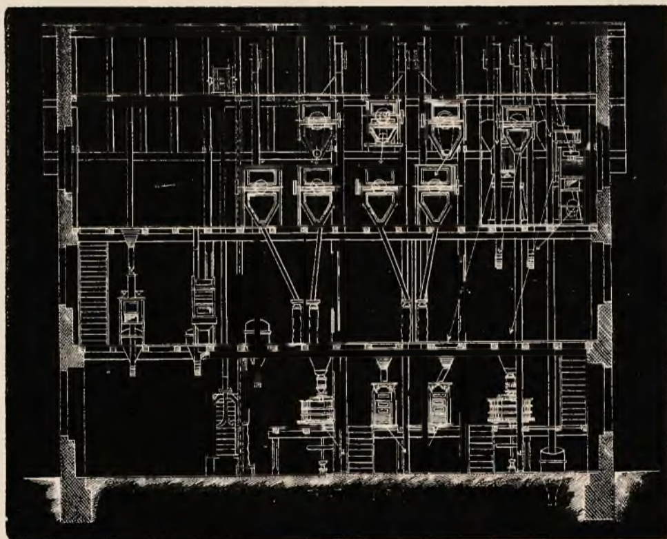
Przekrój podłużny (ryc. 6).
