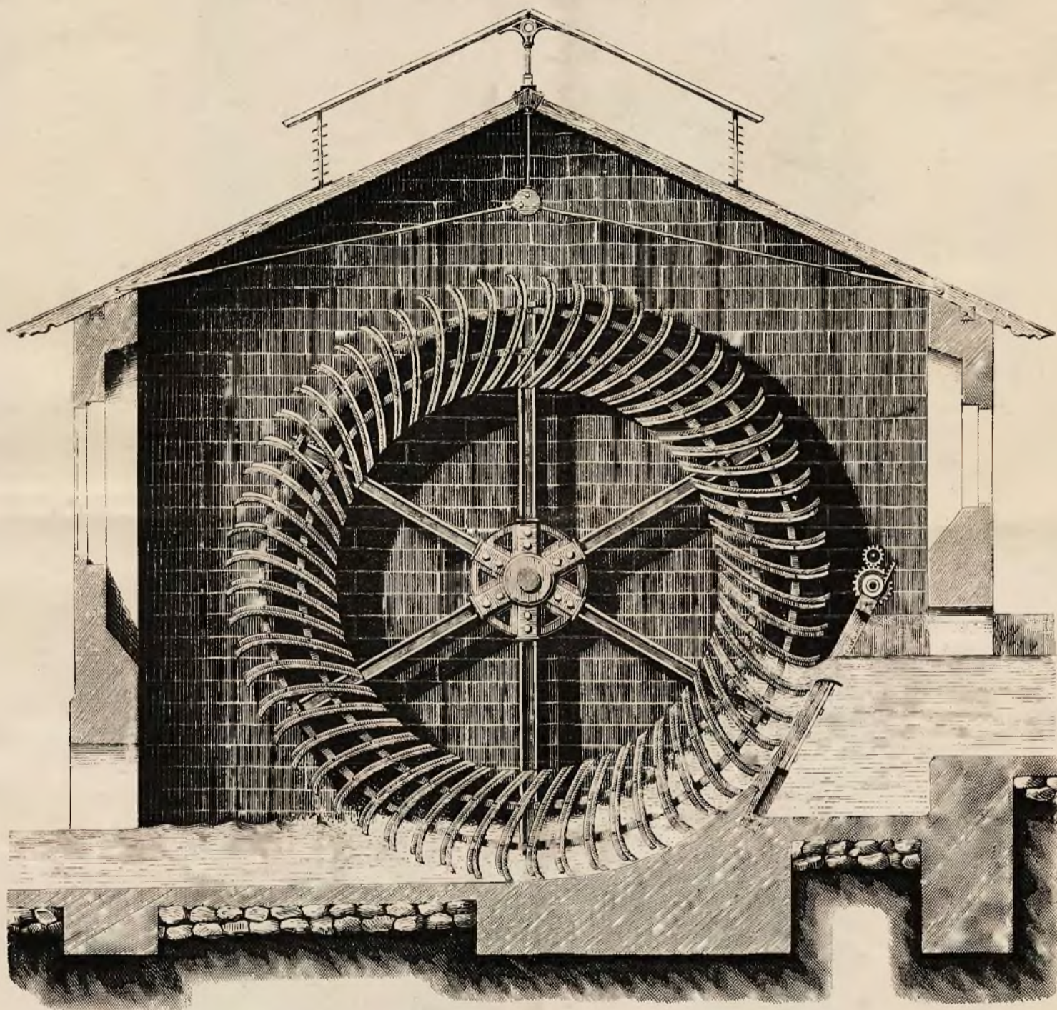
Koło „Sagebien“ (ryc. 4).
