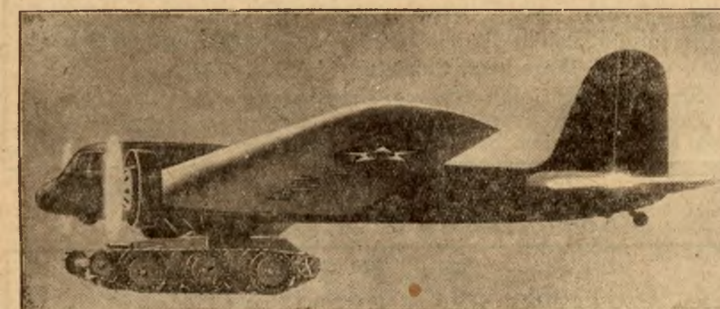
Nowy wynalazek niszczycielski. Model nowego samolotu, połączonego z czołgiem, którego budowę zaaprobowало ministerstwo wojny Stanów Zjednoczonych. Po wylądowaniu samolotu czołg może być odceplony i prowadzić akcję samodzielnie.
