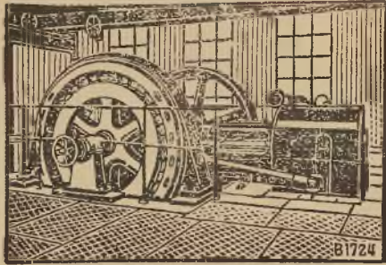
Lanza Lokomobile wentylowa na przegrzaną parę połączona wprost z Dynamo-maszyną.
