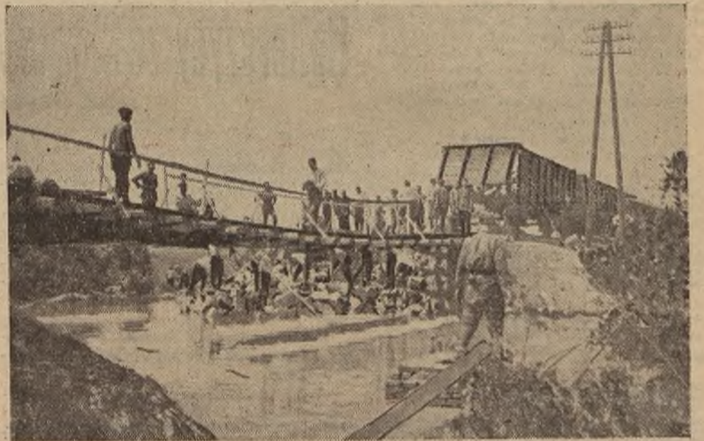
Ilustracja przedstawia wyrwę w nasypie kolejowym koło Biadolin pod Tarnowem. Żołnierze układają kamienie, a na nich spocznie t. zw. prowizorium, które pozwoli przejechać pociągowi.
