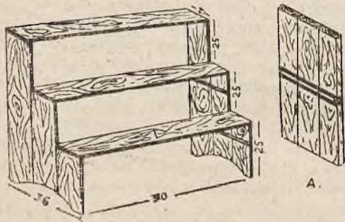
Gėlėms pastatas su trimis lentynomis. Dešinėje (A) parodyta, kaip sujungti lentas.
