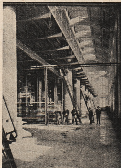
Mościce. Aparatura syntezy amonjaku.
