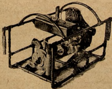
Sikawka motorowa „FLORJANKA” własnej konstrukcji.
