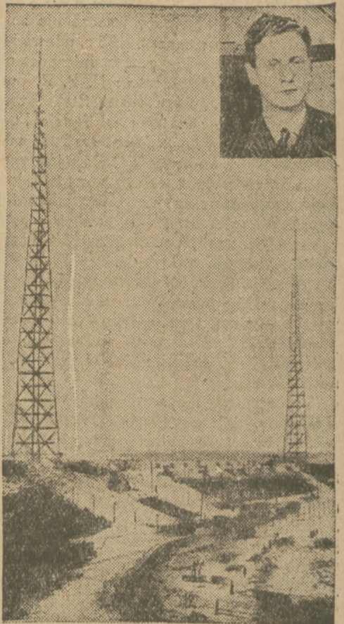
Stacja nadawcza, anteny. U góry kierownik stacji inż. Heller.
