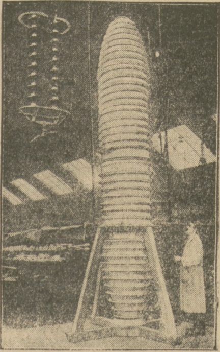
Olbryzi izolator o sile 500.000 volt.
