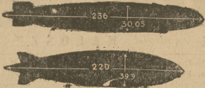
NIEMIECKI ZEPPELIN I ANGIELSKI STEROWIEC „R. 101”
