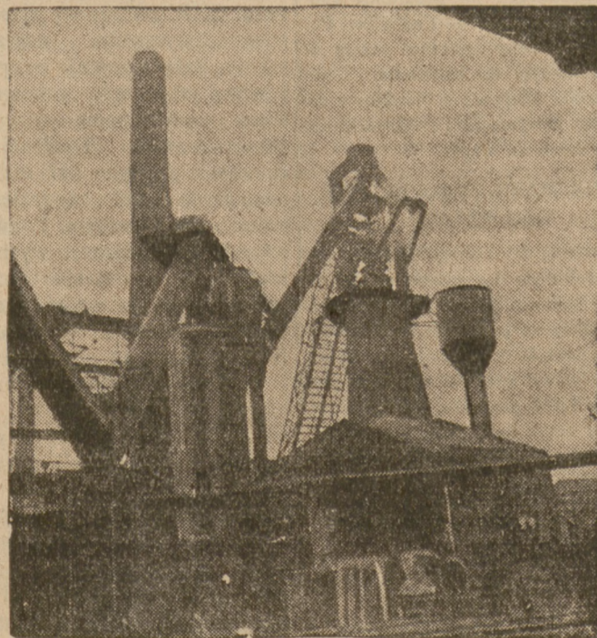
Zdjęcie nasze przedstawia nowo wybudowany wielki piec w hucie „Piłsudski” w Chorzowie, największy w Polsce pod względem wydajności, którego zapalenie odbyło się w tych dniach przy udziale zespołów robotniczych huty.
