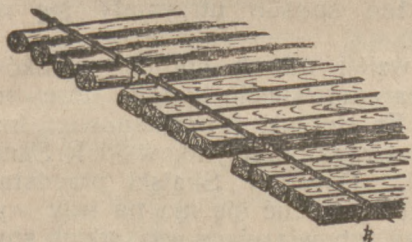
(Rys. 1.) Wiązanie pręgami i wtkami.
