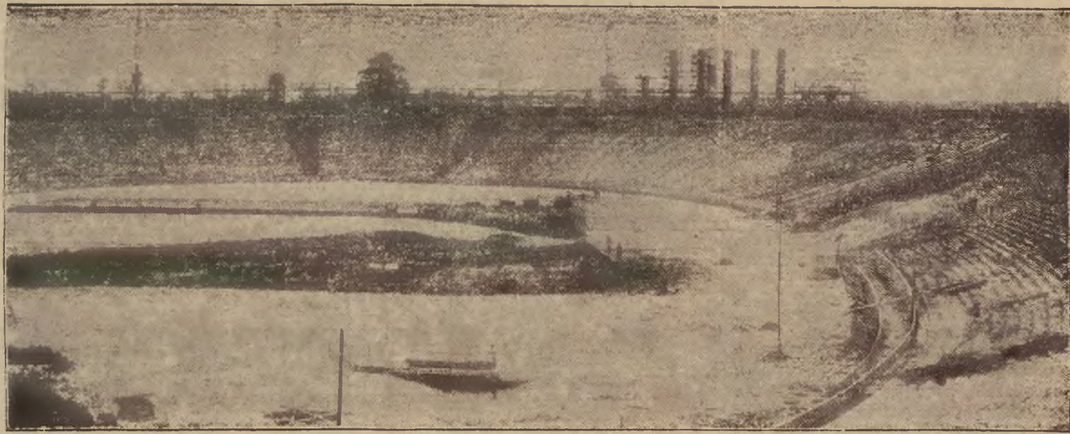
BUDOWA STADJONU OLIMPIJSKIEGO W BERLINIE.
