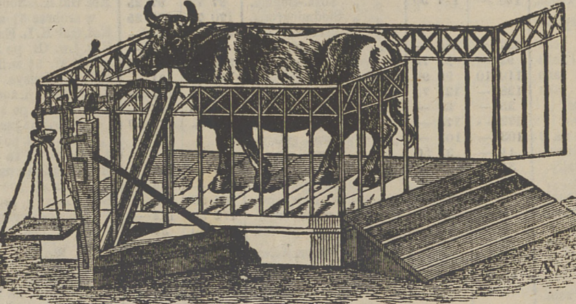
Waga dla bydła z żelaznymi poręczami.
