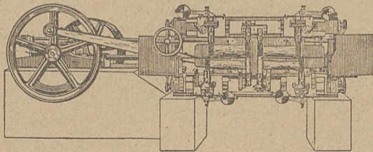
Maszyna do wyrobu wełny drzewnej na 4 drzewa (pnie, belki, bale).
