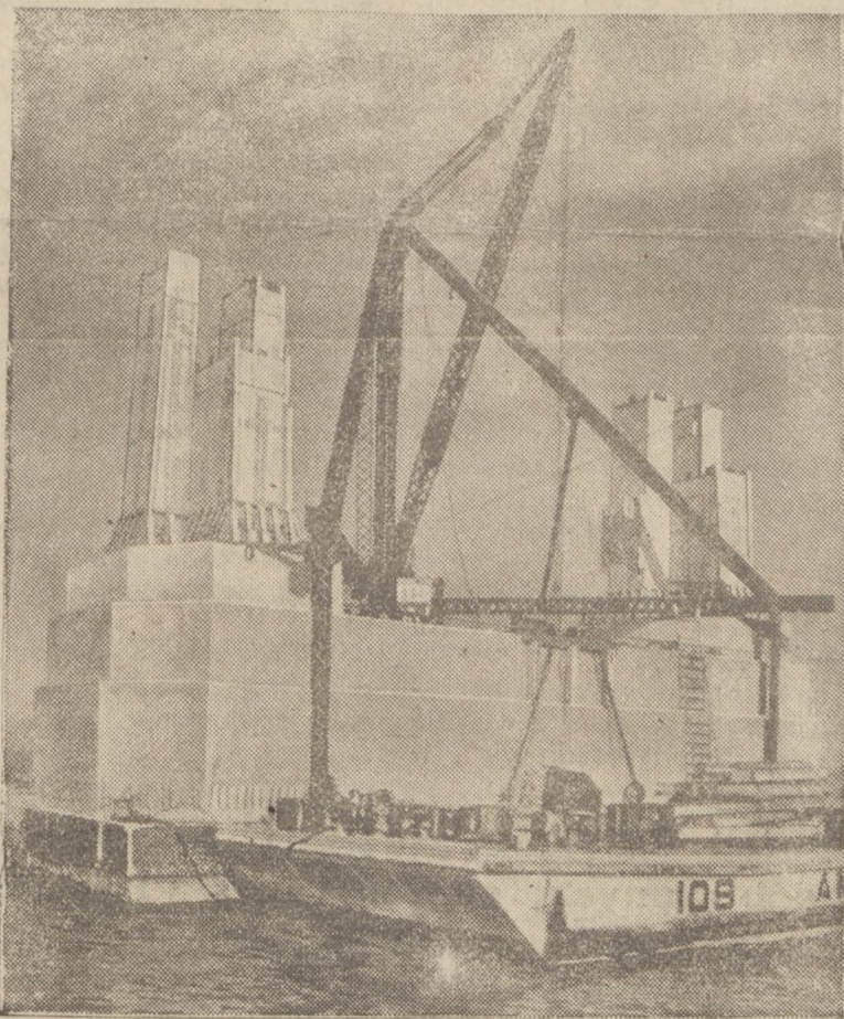
Budowa gigantycznego mostu w Oakland-Bai w pobliżu San Francisco (St. Zjedn.) Uwidocznione na zdjęciu bloki kamienne mają ciężar 10 centnarów każdy.
