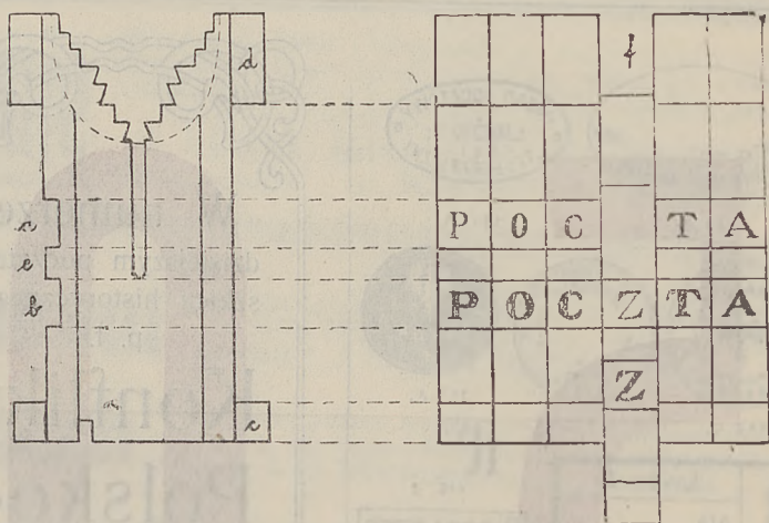
Ryc. 1. Widok matrycy linotypowej z boku i układ słowa „POCZTA“ z cieni- kim „Z“ z uwidocznieniem obsuniętej matrycy. a=wkłębności dla liter cieńskich, b=wkłębności dla liter normalnych, d, c=wystające części matrycy, f=obsunięta matryca litery „Z“.
