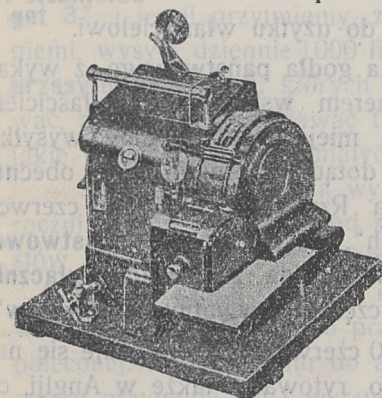
Automat do drukowania znaczków pocztowych — „Midget 3“, przyjęty przez nasze M. P. i T.
