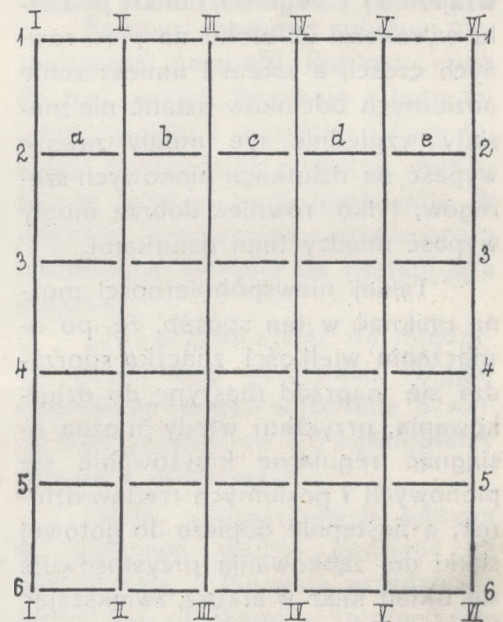
Ryc. 4. Układ sztańc do dziurkowania jednego 25-bloku t. j. 1/4 arkusza I. — VI jednolite, pionowe szeregi sztańc, 1—6 szeregi poziome złożone z odcinków a, b, c, d, e, zawierających po 10 sztańc.
