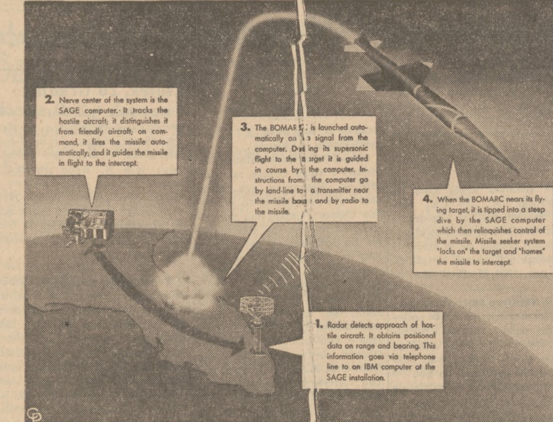
JAK WYGLĄDA OBRONA PRZECIW ATAKOM Z POWIETRZA. — Rysunek powyższy daje ogólny obraz, jak wygląda dziś system obrony kraju od ataków z powietrza. Nadlot nieprzyjacielskiego obiektu alarmowany jest i wysłany przez urząd radarowy. Sąd przekazane zostaje do systemu kontrolnego "Sage" (w górze — w lewo). Sąd na stopie odpalenie rakiety "Bomarc", która automatycznie ściga obiekt aż do zniszczenia go. System w zadenie nie musi być scentralizowany, n.p. odalenie następuje w Cape Canaveral a system kontrolny i uruchamiający odalenie jest w Kingstown, N. Y.
