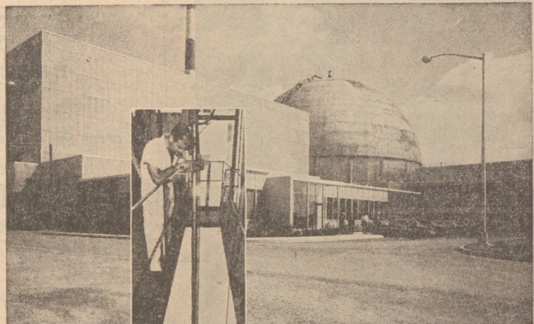
Na stacji Commonwealth Edison Co. w Dresden, w pobliżu Morris, Ill., uzyskano w czwartek pierwszy sukces w zapaleniu pierwiastka promiennego — uranum, umieszczonego w reaktorze znajdującym się pośrodku 190-stopowego pieca stalowego.
