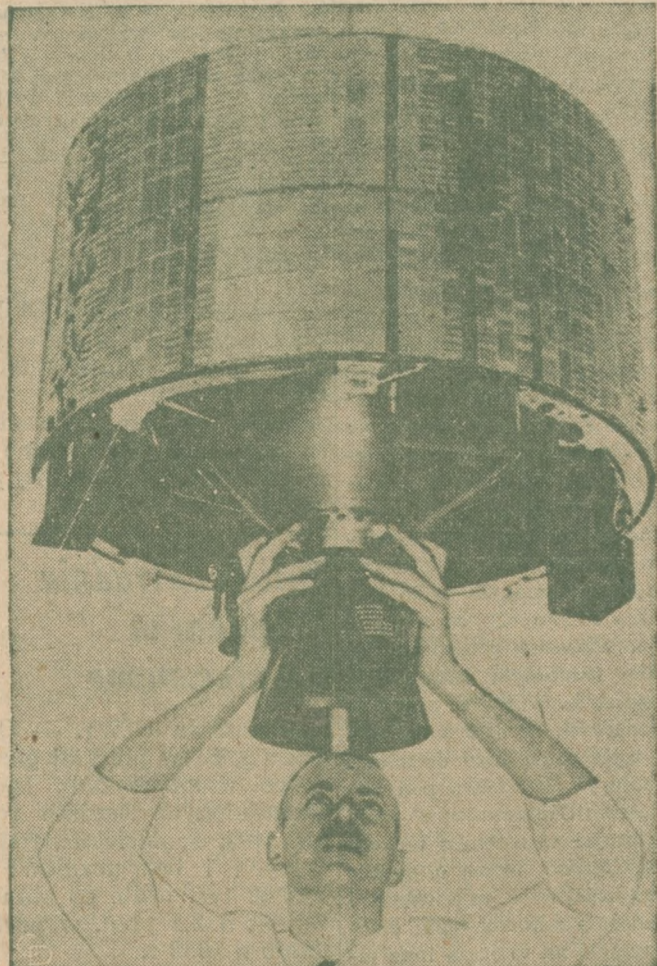
SATELITA NIERUCHOMY — Jeden z techników (powyżej) dokonuje w Cape Canaveral, na Florydzie końcowych poprawek na instrumencie "Syncom", satelity nieruchomego — przed wysłaniem tego aparatu, planowanego na 6-go lutego. Poprawki polegają na tym, by nadać mechanizmowi rotacyjnemu Syncom'u na wysokość 22,300 mil taką samą szybkość co posiada Ziemia. Przez co "Syncom" będzie jakby "stał" nieruchomo w powietrzu, mimo swego obrotu.
