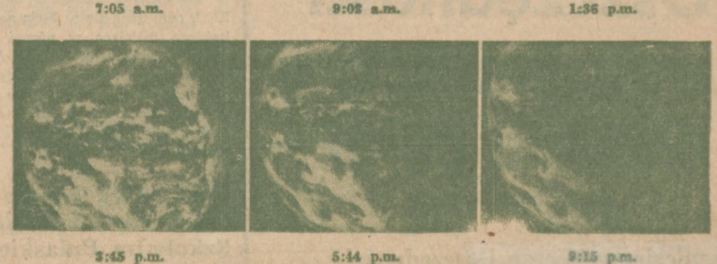
SATELITA "APPLICATIONS TECHNOLOGY" przysiał z wysokości 22,300 mil w przestrzeni powyższe zdjęcia ziemi wskazujące zmiany w układzie chmur w ciągu 14 godzin.
