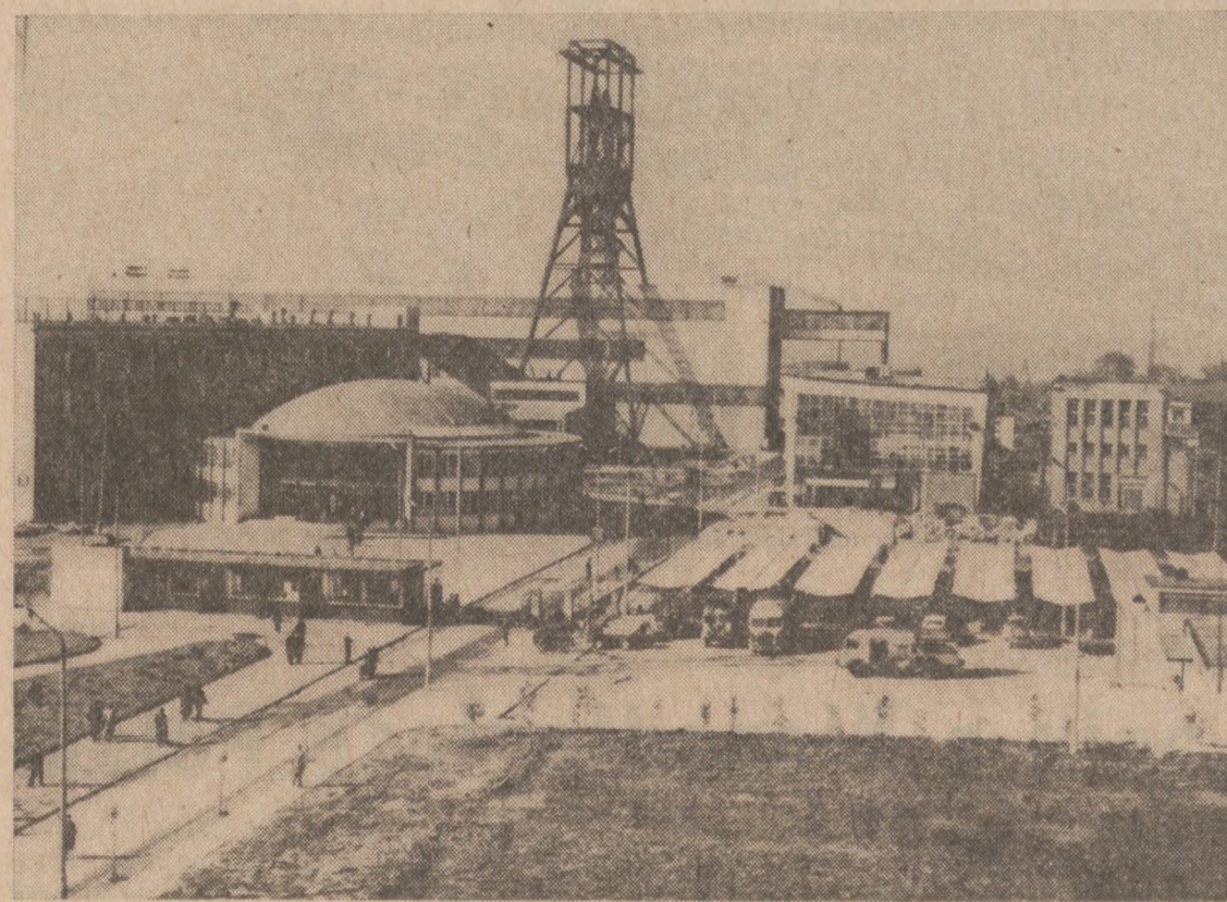
Nowa kopalnia węgla "Jastrzębie" w Rybnickim Okręgu Górniczym.
