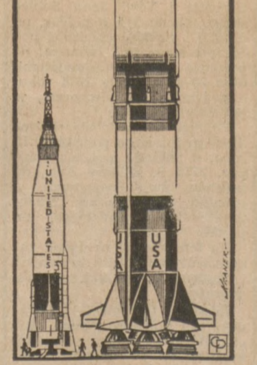
NA ZDJĘCIU: pierwszy amerykański załogowy pojazd kosmiczny Mercury Redstone (po lewej), na którego pokładzie w maju 1961, Alan Shepard, jako pierwszy amerykański astronauta, odbył podróż w przestrzeń. Po prawej — statek kosmiczny Apollo 14, którego kapitanem załogi jest Alan Shepard. Redstone liczył zaledwie 94 stopy długości podczas gdy wysokość Apollo 14 wynosi 364.
