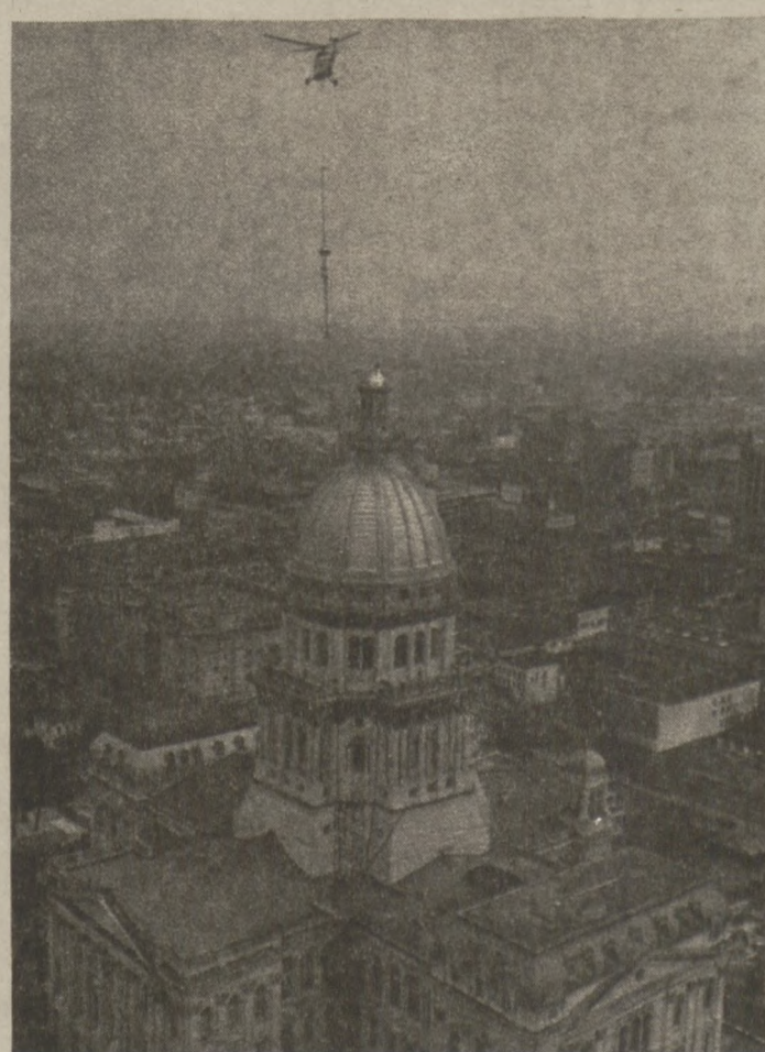
SPRINGFIELD, ILL. — Specjalna ekipa robotników, przy użyciu helikoptera, zakłada nowy maszt na Kapitolu stanowym. Stalowa iglica liczy 63 stopy długości. (UPI)
