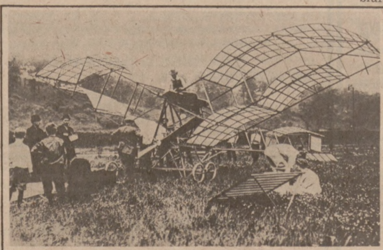
Maszyna Latająca Zaprojektowana Przez Polskiego Mechanika, Pensylwania, 1910.
