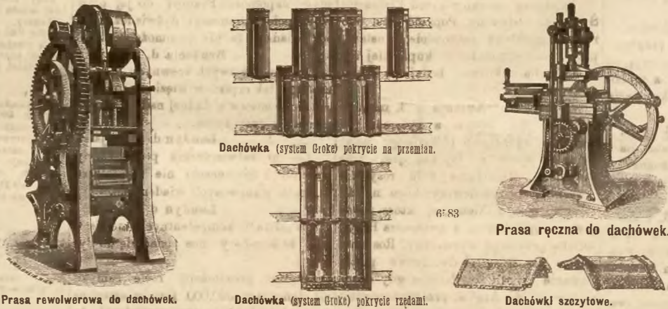
Prasa rewolwerowa do dachówek. Dachówka (system Groke) pokrycie na przemian. Prasa ręczna do dachówek. Dachówka (system Groke) pokrycie rzędami. Dachówki szczytowe.
