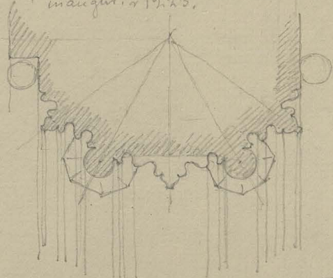
Krój rzyt skłepienia wspanionoy.
