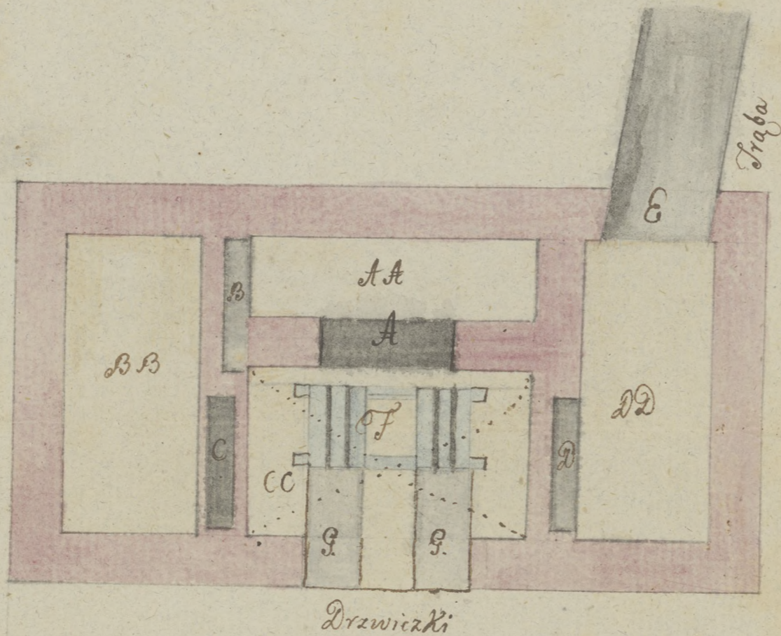
Fundament Pieca.
