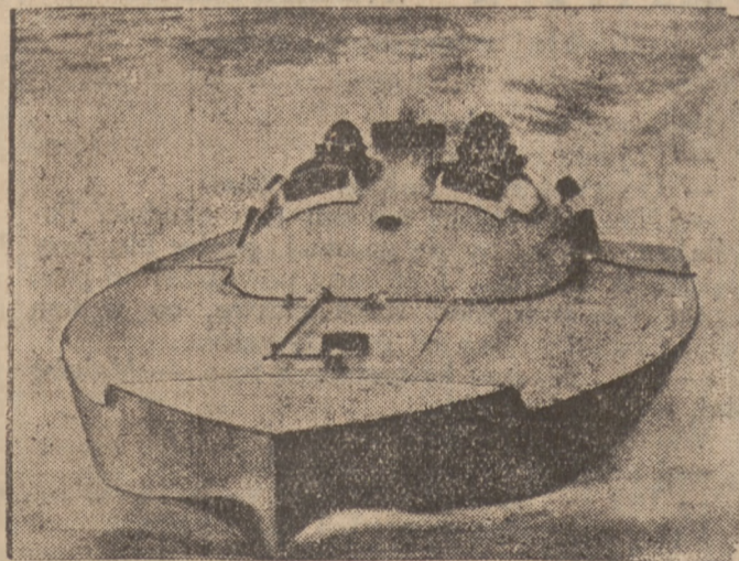
Angielska łódź motorowa „Miss Britoin III” osiągnęła w Southampton na morzu nowy rekord szybkości 161,5 klm. na godzinę.
