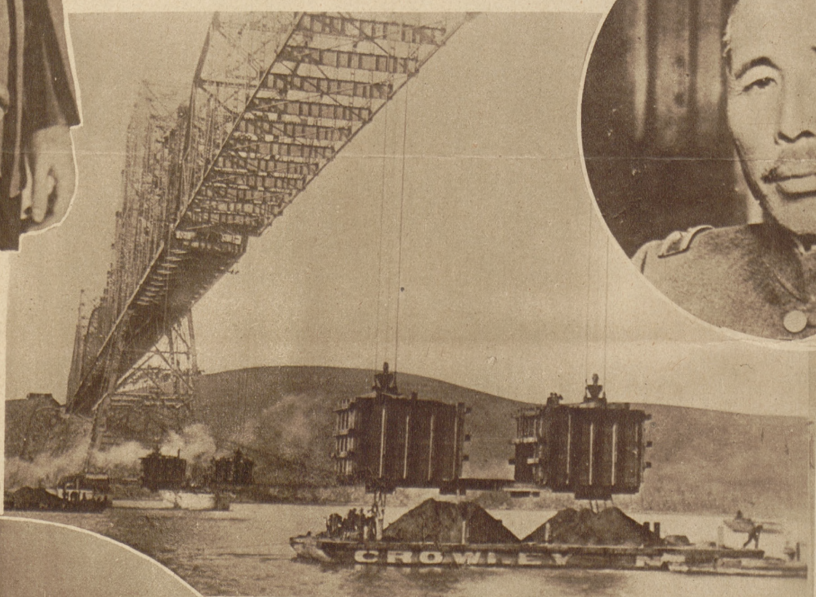
U dołu: Z budowy olbrzymiego mostu w Carquinez Straits (St. Zjedn.). Potężne tuki mostu dla przeciwwagi obciążone są od dołu wagonami z piaskiem, które się w odpowiednim momencie opróżnia.
