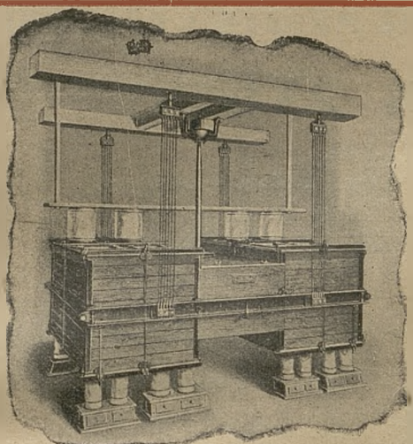
Planzychter 4-działowy
