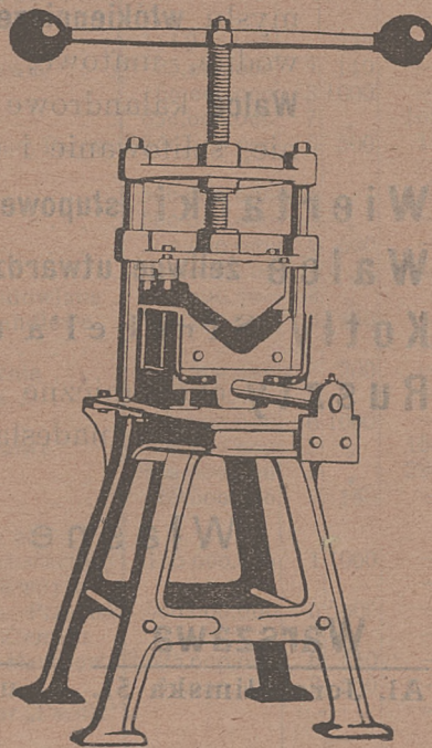
Ręczna Prasa do dachówek i gąsiorów na glinę.
