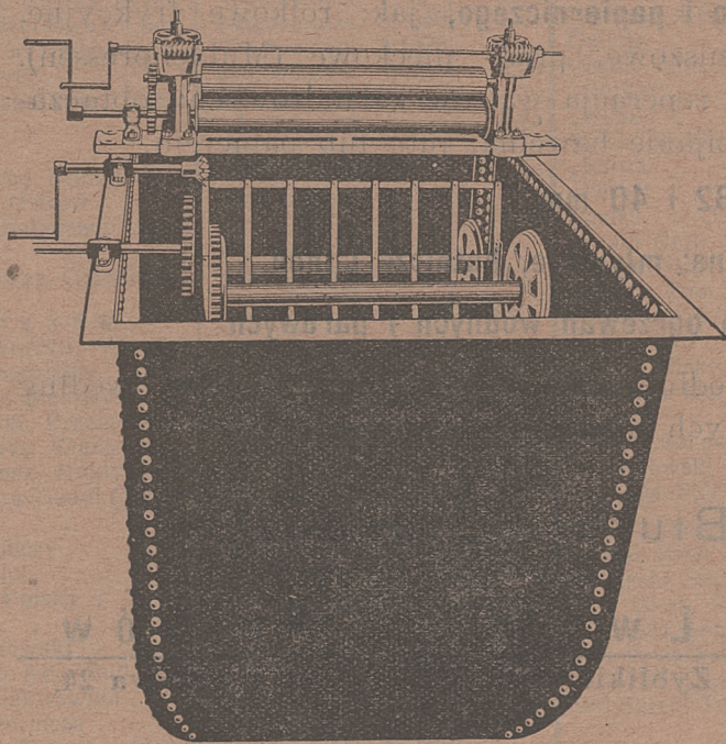
Mechaniczna Maszyna do produkcji papy dachowej.
