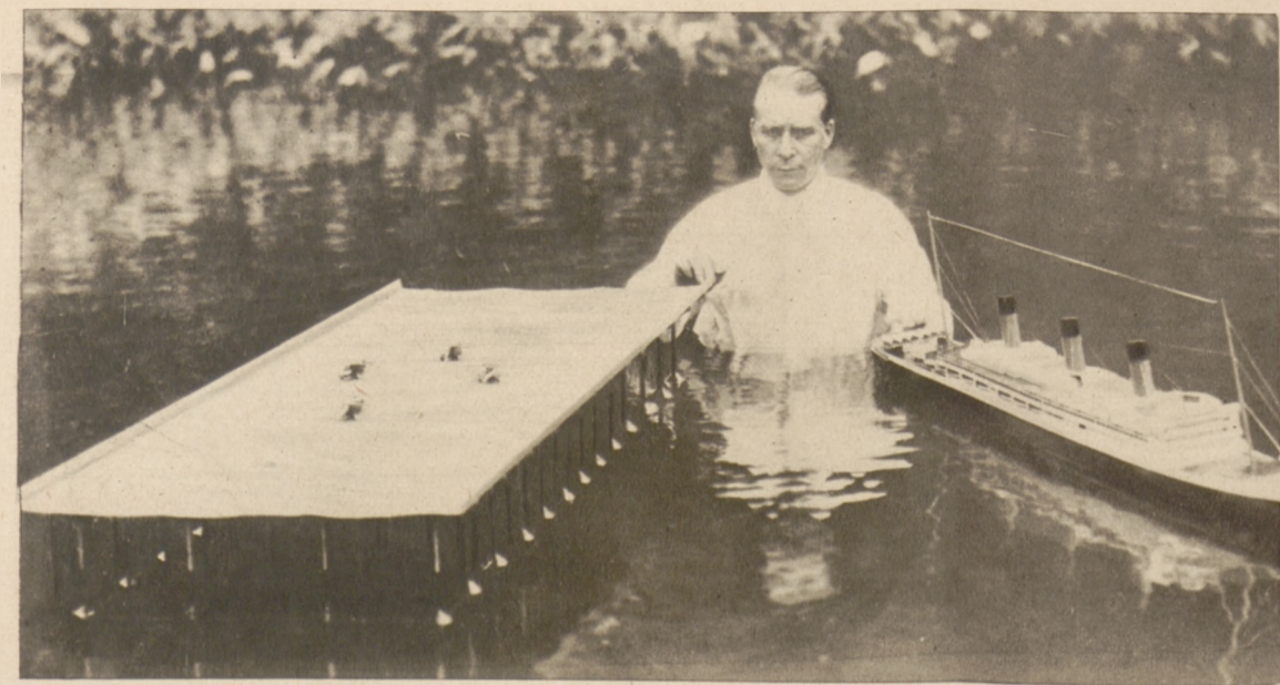
Amerykański inżynier Armstrong pracuje nad skonstruowaniem pływającej wyspy stalowej przeznaczonej do lądowania na niej samolotów transoceanicznych między Ameryką a Europą. Na zdjęciu widzimy Armstronga, robiącego doświadczenia z modelem wyspy na wodzie. Dla porównania obok zmniejszony model okrętu Majestic.
