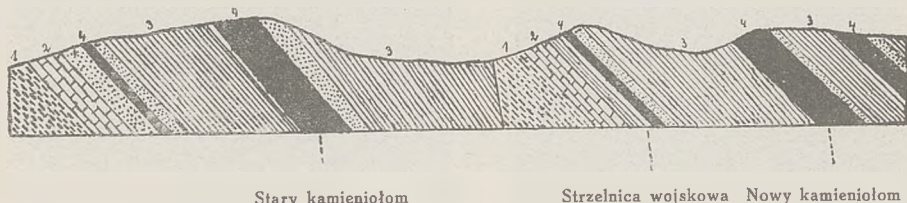
3. Przekrój wzdłuż prawych stoków doliny Olzy (według Uhliga).
