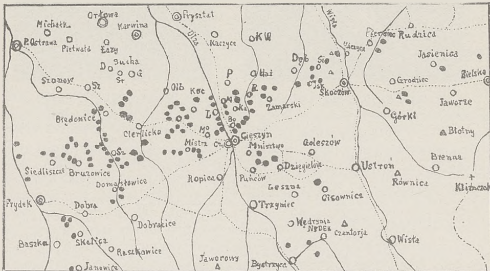
6. Znaczenie cieszynitów na Śląsku Ciesz.; czarne kropki oznaczają odkrywki cieszynitów; według mapy prof. Kazimierza Smulikowskiego.
