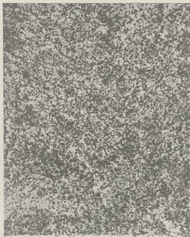
4. Typowy okaz drobnodziarnistego cieszyńszynu w naturalnej wielkości (z Puńcowa); szlif. prof. Kazimierza Smulikowskiego.
