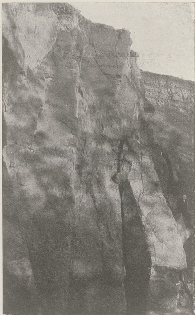
1. Kamieniołom cieszynitu w górnej części w Boguszowicach; na prawo u góry widać warstwy górnych łupków cieszyńskich. Fot. A. Błahut, Cieszyn.
