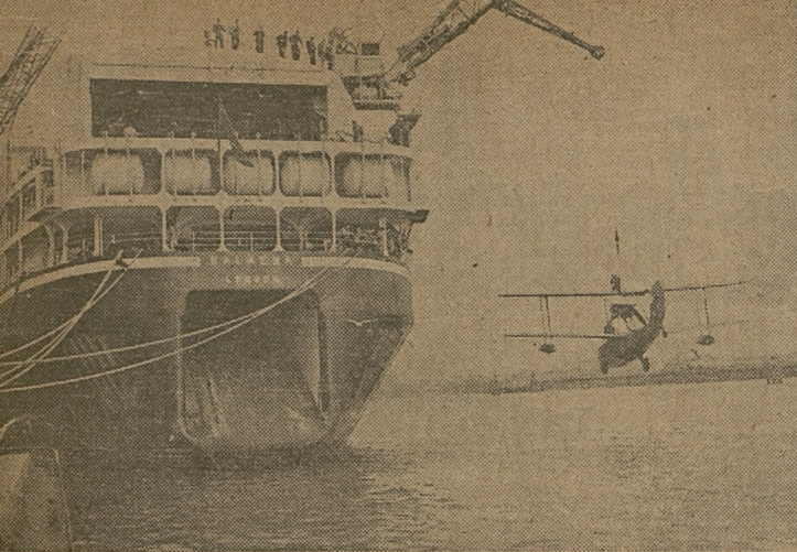
Statek - fabryka wielorybnicza. Widok od rufy. Widoczny otwór do wyciągania wielorybów na pokład oraz samolot wywiadowczy
